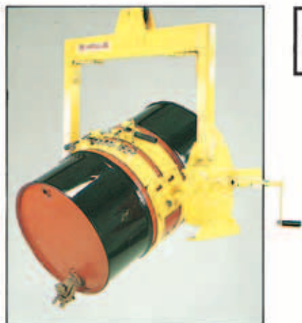
Mod. DTU/HD/H/DG/CH. Versione pesante. Ribaltamento del fusto tramite riduttore comandato da manovella o catena di comando.
