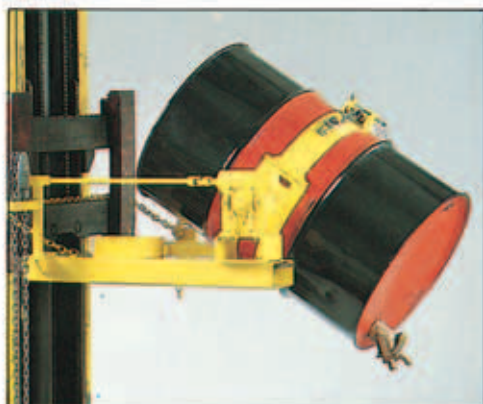
Mod. DTU/F/DG/CH. Per ribaltare e travasare agevolmente i vostri fusti a qualsiasi altezza utilizzando il vostro carrello elevatore. Comandi a manovella o tramite catena.
